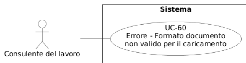
Figura 97: Diagramma del caso d'uso UC-60: Errore per formato documento non valido per il caricamento
